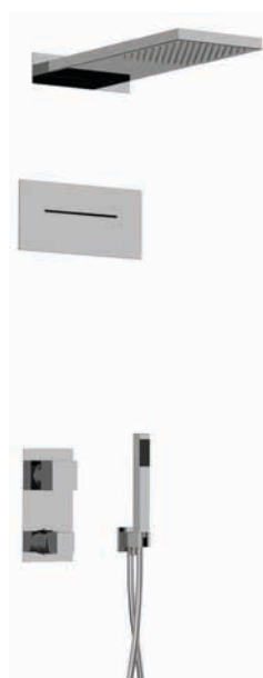
17BRIP3SR002 Set doccia composto da: miscelatore a incasso con deviatore a 3 vie (173RIP3); soffione a parete 50x20 cm con getto a pioggia, in acciaio INOX lucidato (SR002); doccetta minimale quadrata a 1 funzione, in ottone (191PF); presa acqua con supporto fisso (242PA); bocca a cascata ad incasso 14,5x30 cm (13BBC); flessibile 150 cm. Shower set including: built-in mixer with 3-way diverter (173RIP3); 50x20 cm wall shower head with rain jet, in polished stainless steel (SR002); 1-function squared hand shower, in brass (191PF); brass connection pipe with shower holder (242PA); built-in waterfall spout, 14,5x30 cm (13BBC); 150 cm flexible hose. CR
